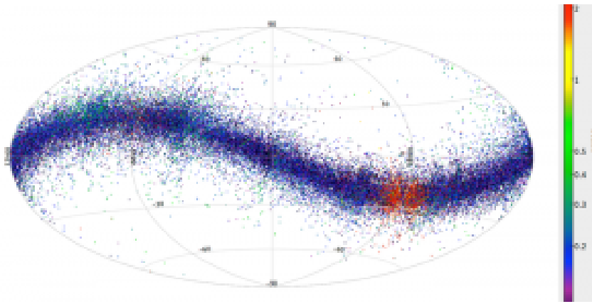
Gaia's asteroid detections. ESA/Gaia/DPAC/CU4, L. Galluccio, F. Mignard, P. Tanga (Observatoire de la Côte d'Azur)
